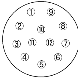
12ピン(オス)
